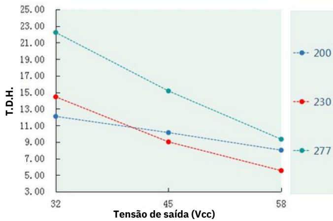
T.D.H. x Tensão de saída (DL-100H-MAL)
