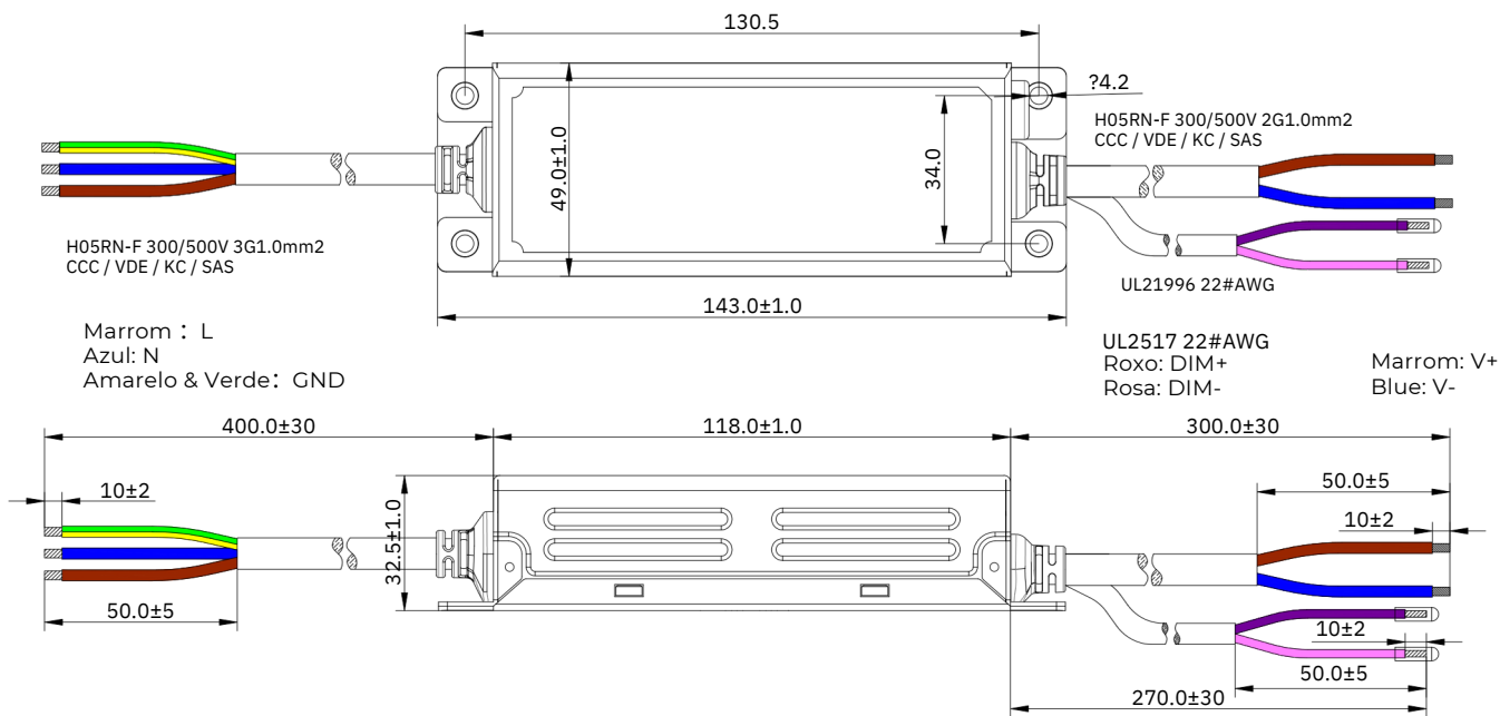
Desenho dimencional DL-100H-58S-MAL
