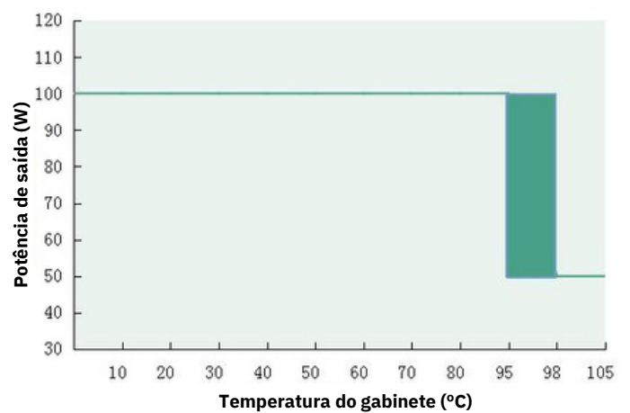
Potência de saída x Tgabinete (DL-100H-MAL)
