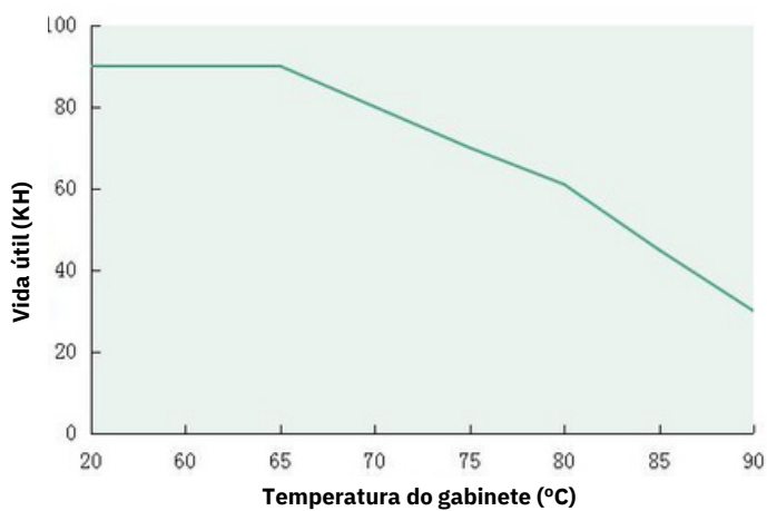
Tgabinete x Vida útil (DL-100H-MAL)
