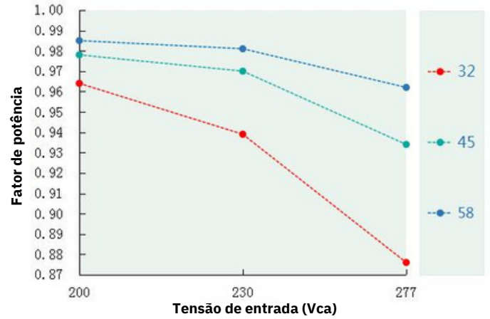
Fator de potência x Tensão de entrada (DL-100H-MAL)
