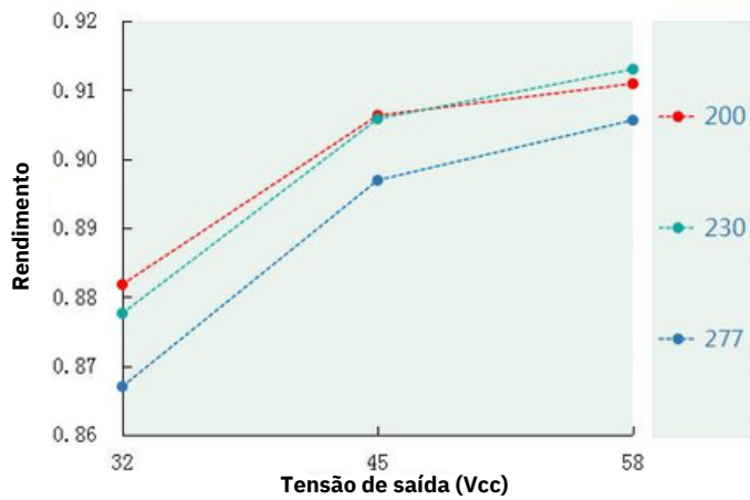
Rendimento x Tensão de saída (DL-100H-MAL)
