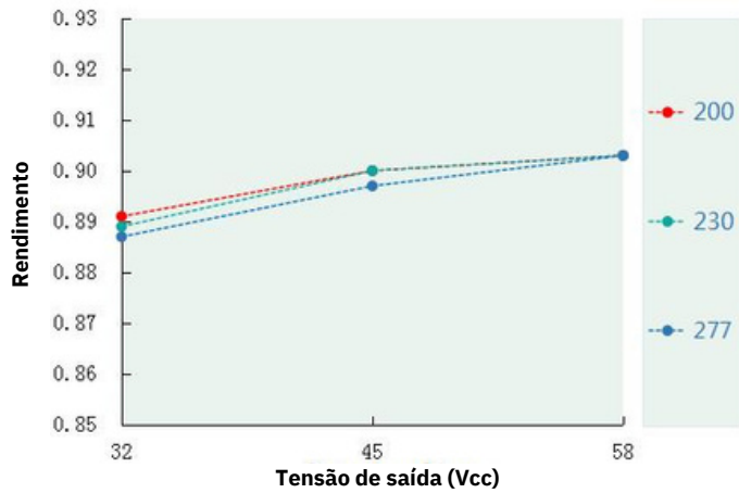
Rendimento x Tensão de saída (DL-75H-MAL)
