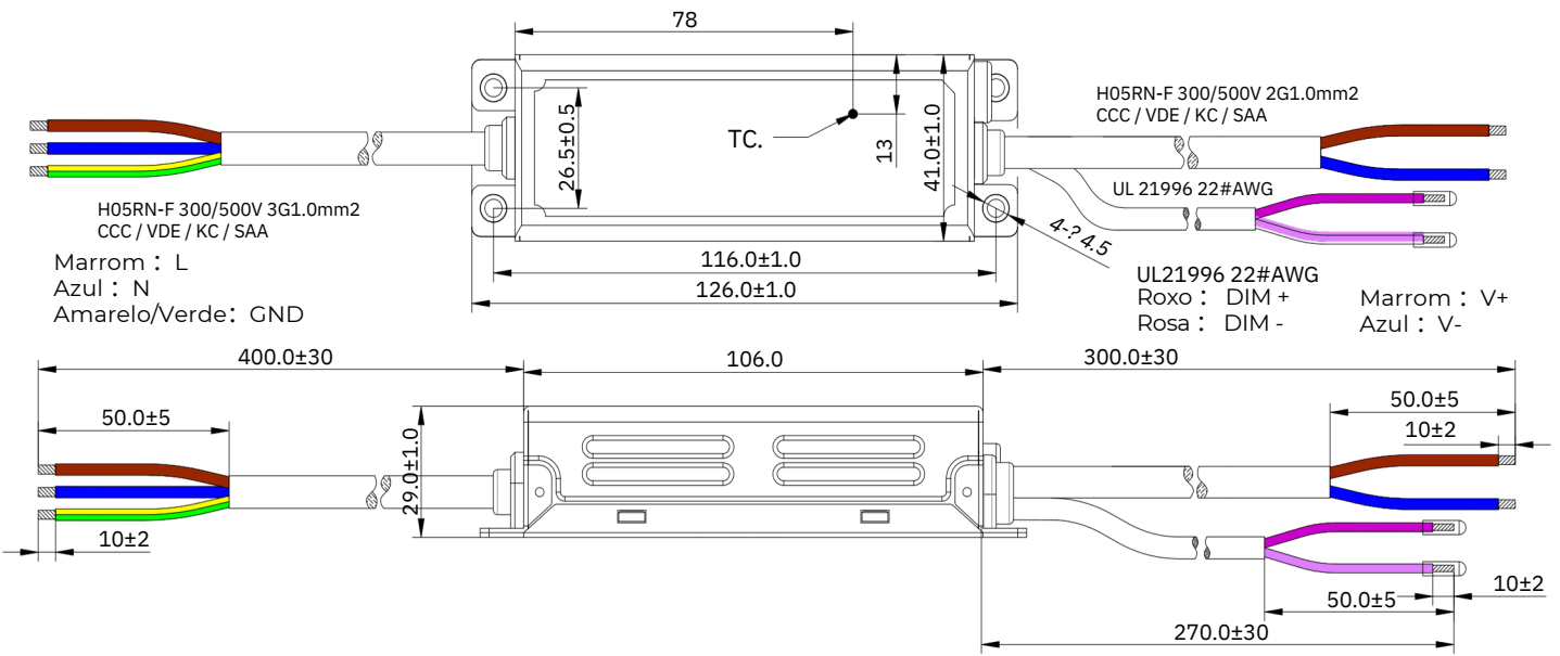
Desenho dimencional DL-75H-58S-MAL
